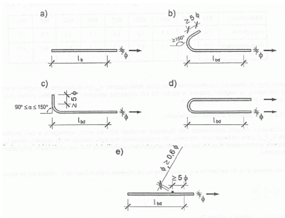
Rysunek 45 – Obliczeniowe długości zakotwienia; a) zakotwienie proste, b) hak półokrągły, c) hak prosty, d) pętla, e) przypojonny pręt poprzeczny
